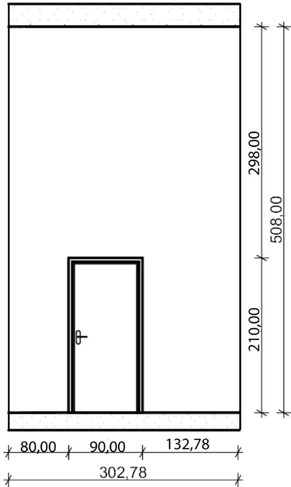
B NÉZET
