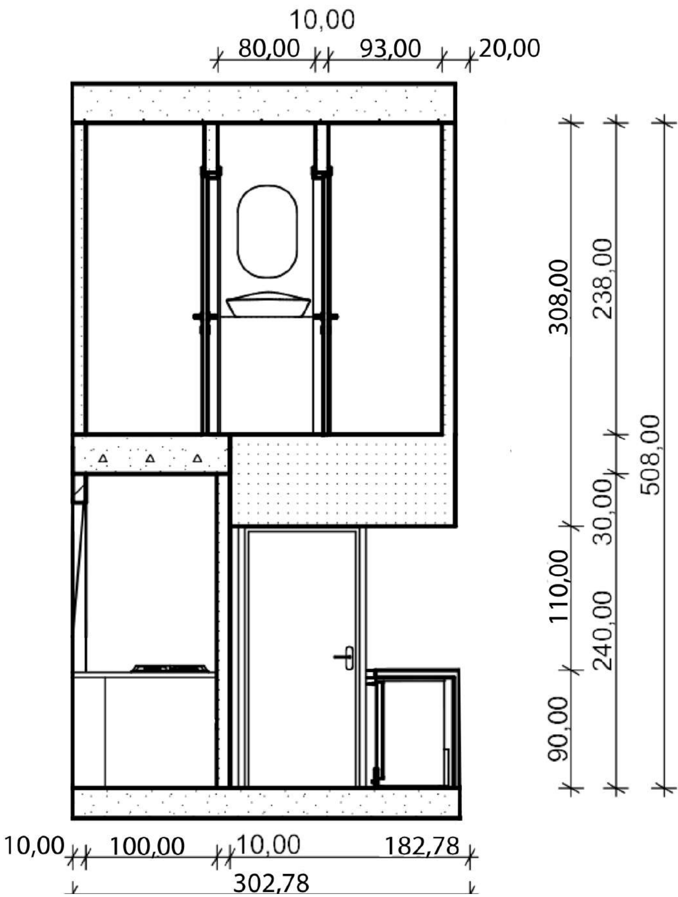
C METSZET
